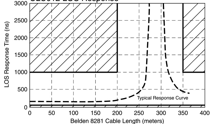
CLC012 LOS Response
