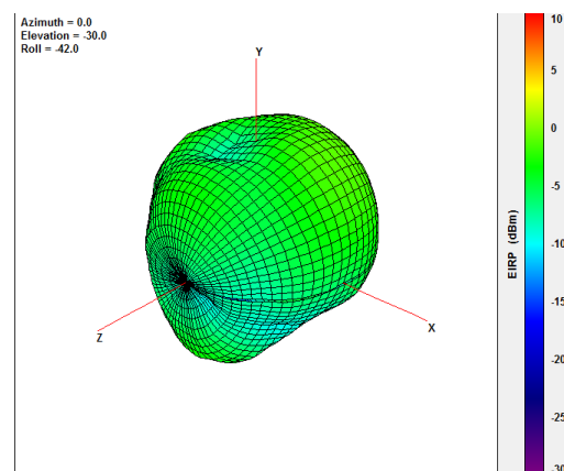
@960MHz
