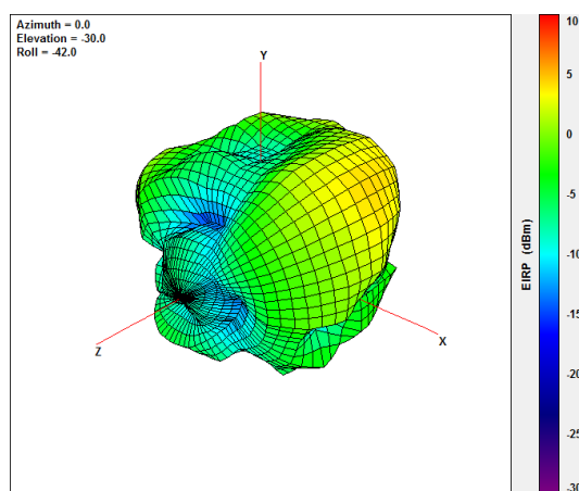
@2690MHz
