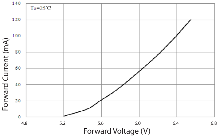
V_f ----- I_f
