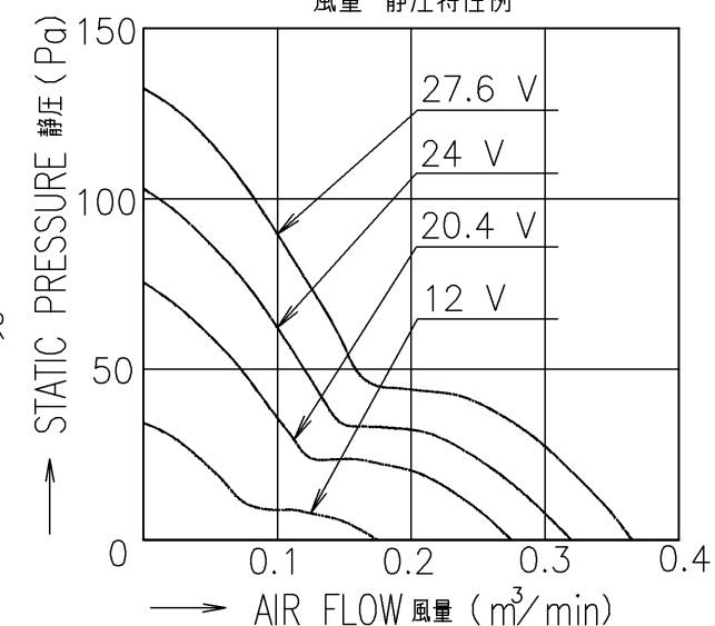
風量-靜圧特性例
