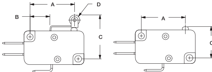
FIG. 1 Lever Roller
