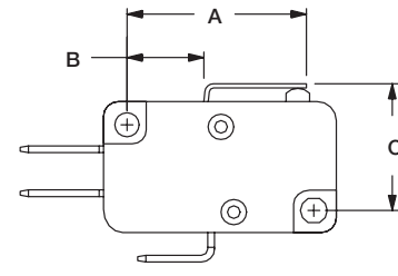
FIG. 3 Lever
