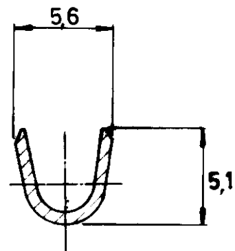
SECCION C C
