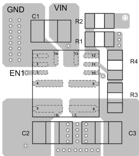
Top Layer
