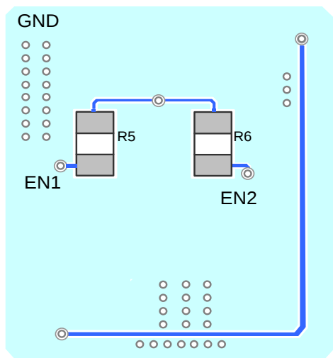
Bottom Layer
