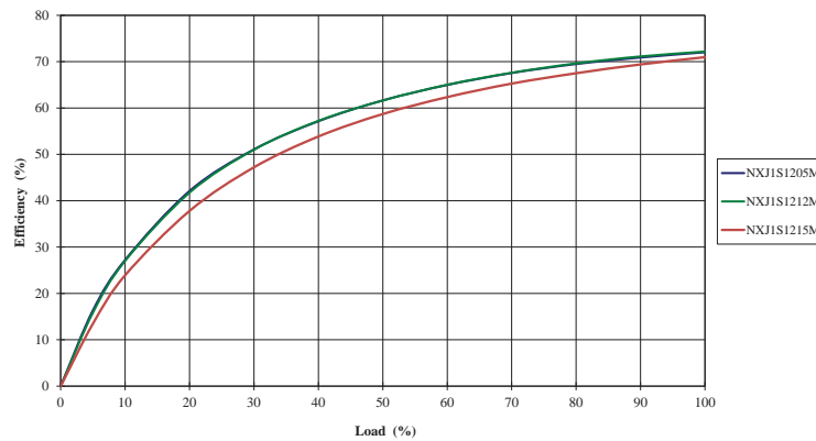
12V Input
