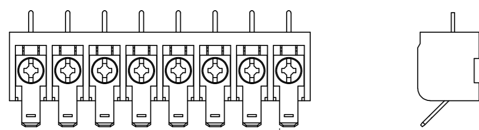
796905-1 .187 TYP
