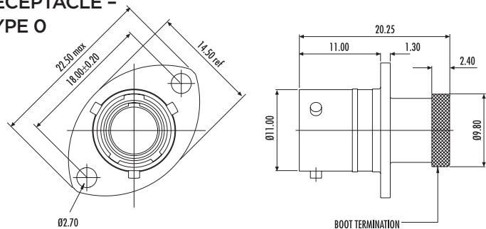
HERMETIC RECEPTACLE
