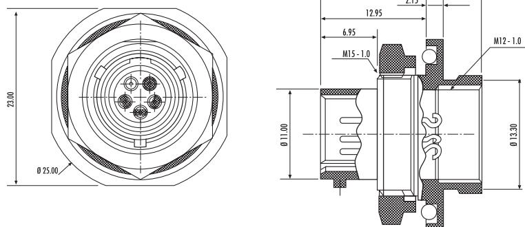
HERMETIC RECEPTACLE
