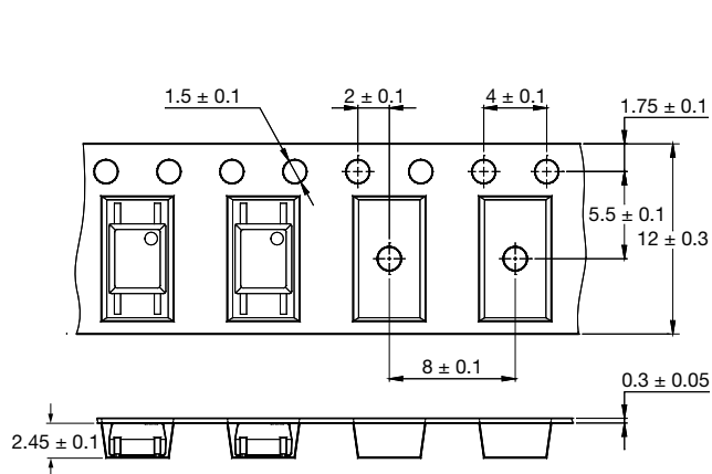
Fig. 18 - Tape Dimensions
