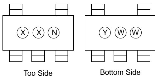
5-Pin SC-70/SC-70R
