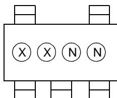
5-Pin SC-70/SC-70R
