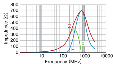
MMZ1608D301BTD25
