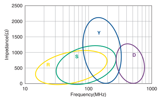
MMZ2012 Type
