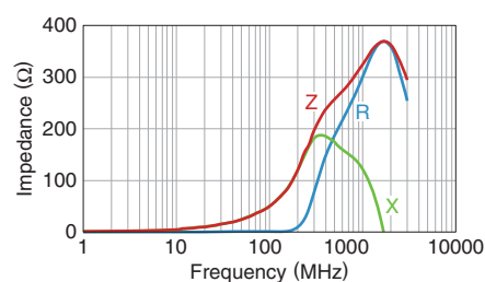
MMZ1608D121CTDH5
