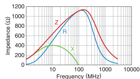
MMZ1608R600ATD25
