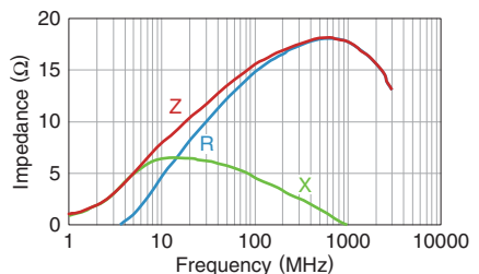
MMZ1608R121ATD25
