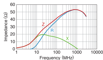
MMZ1608S400ATD25
