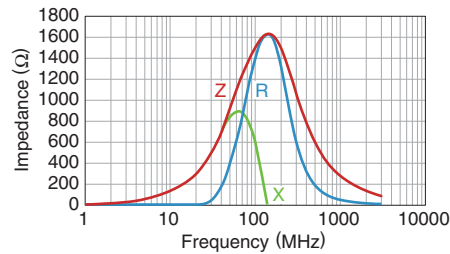
MMZ1005D220CTD25
