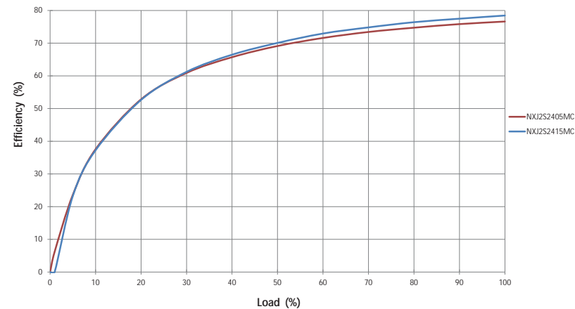
24V Input
