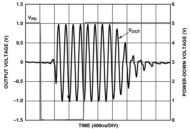
Figure 27. Enable/Power-Down Time
