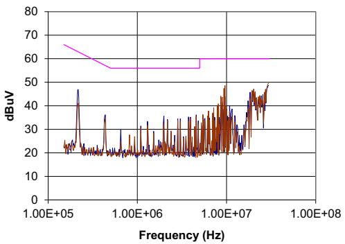
NCS12S1212C
