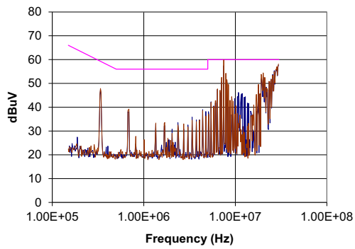
NCS12S4815C
