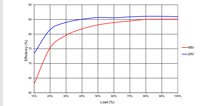
NCS12S4815C
