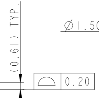
SCALE 4:1
