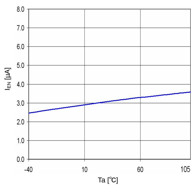
Fig.24 T_a - I_{EN}
