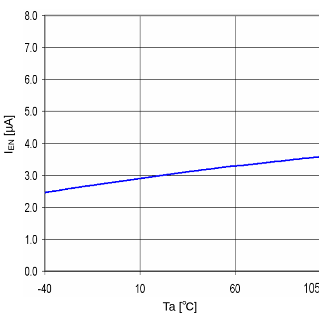
Fig.24 T_a - I_{EN}
