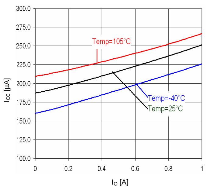
Fig.32 Io-Icc
