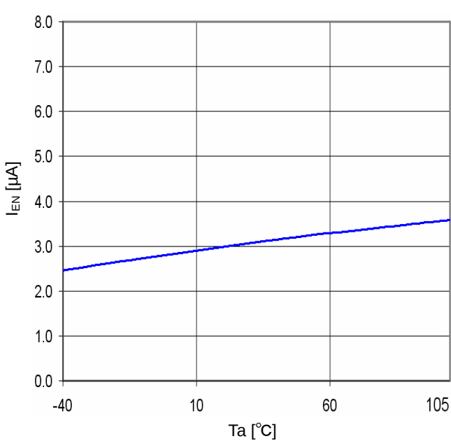
Fig.24 T_a - I_{EN}
