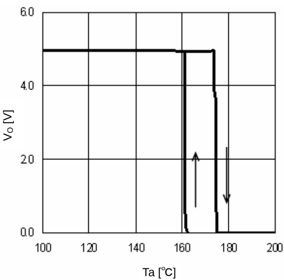
Fig.28 TSD ( I_o=0\text{mA} )
