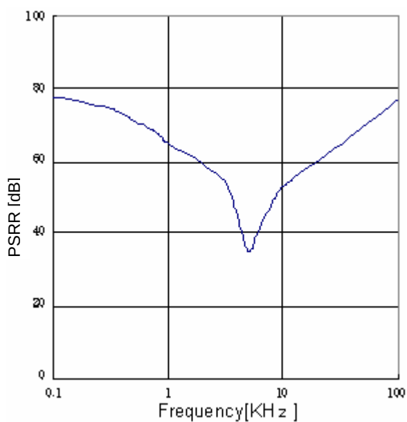
Fig.33 PSRR (Io=0mA)
