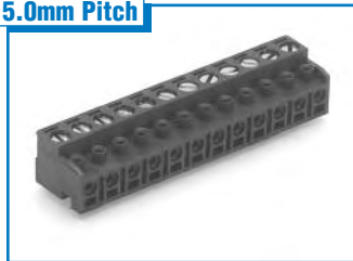
ESZP Compact . . . . . Page 37 12A / 250V
