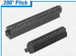
ELFK 45° Angle . . . . . Page 39 ELFK w/ Locking Ears . . . . Page 41 15A / 300V
