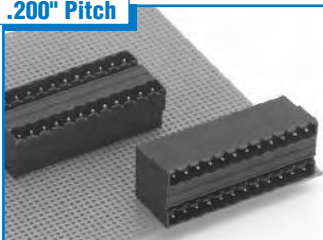
ELFA 2-Tier Aligned H/V . . . Page 49 15A / 300V
