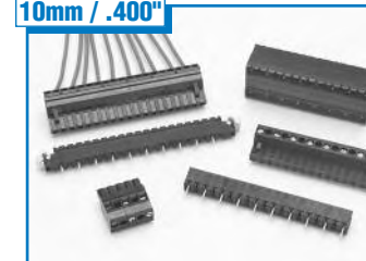
10mm / .400"
