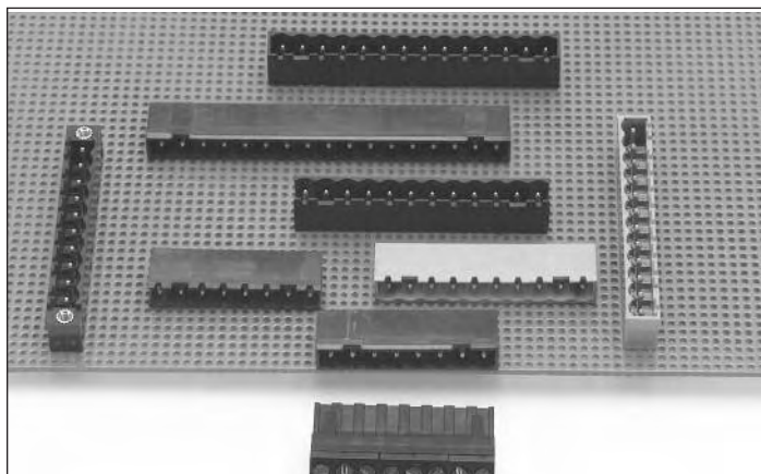
ELFH Horizontal—Eared
