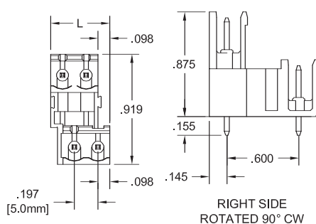
ELFD—Vertical
