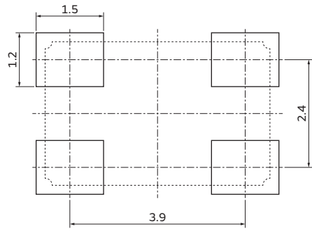
XRCLK (TSS-5032A)
