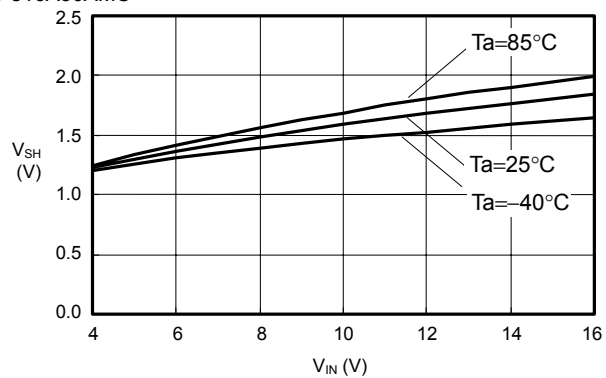
V_{IN}-V_{SH} S-816A30AMC
