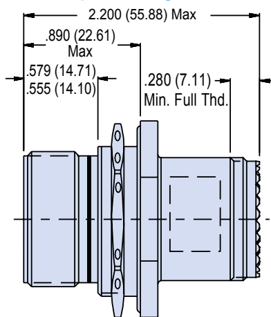
Jam Nut
