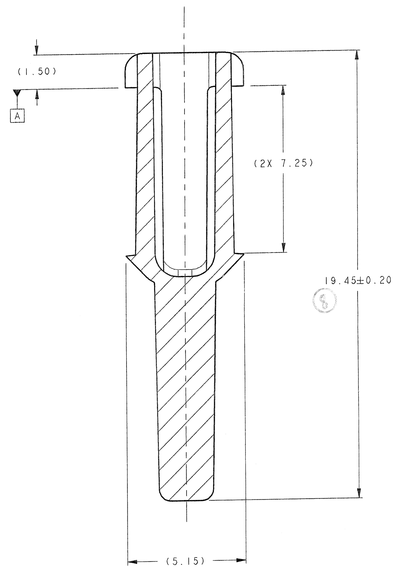
SECTION A-A
