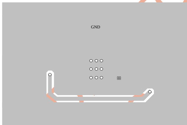
Bottom Layer
