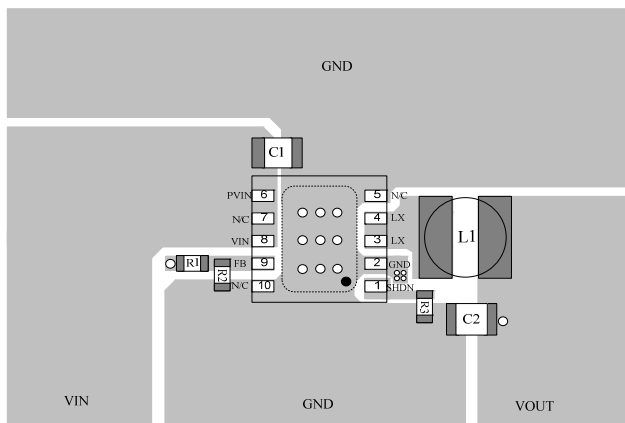
Top Layer
