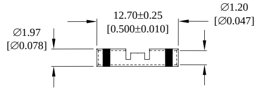
5) CRIMP SPLICE, Qty.: 2
