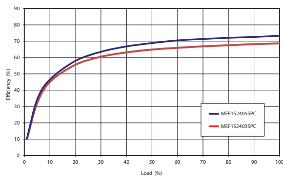
24V Input
