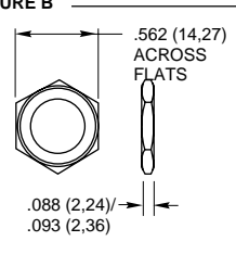
Hex Nut
