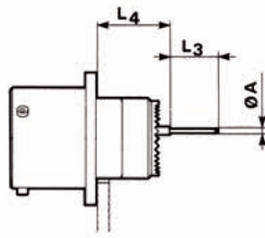
Receptacle type 0
