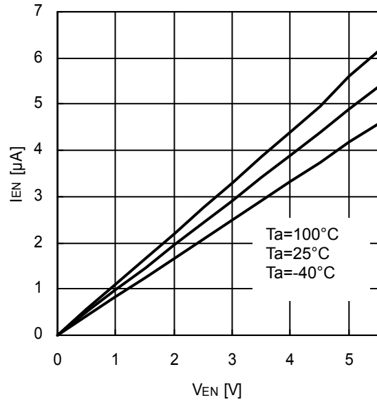
Figure.14 V EN -I EN
