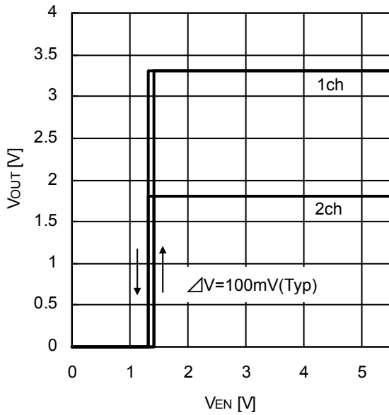
Figure.13 V EN -V OUT
