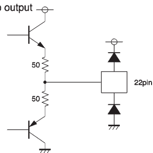
Op-amp output
