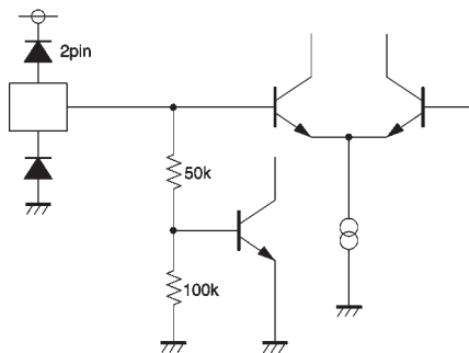
Op-amp input
