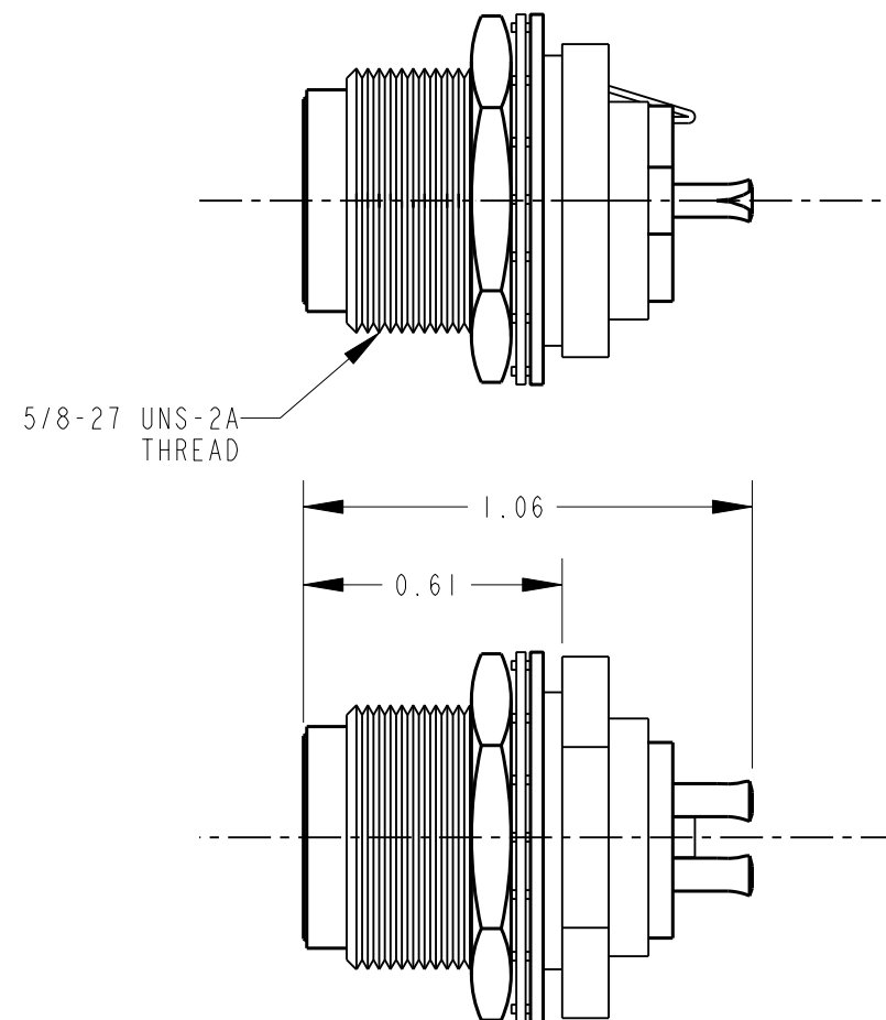
SL173MX 3PIN
