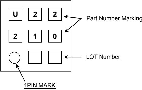
VQFN016V3030(TOP VIEW)
