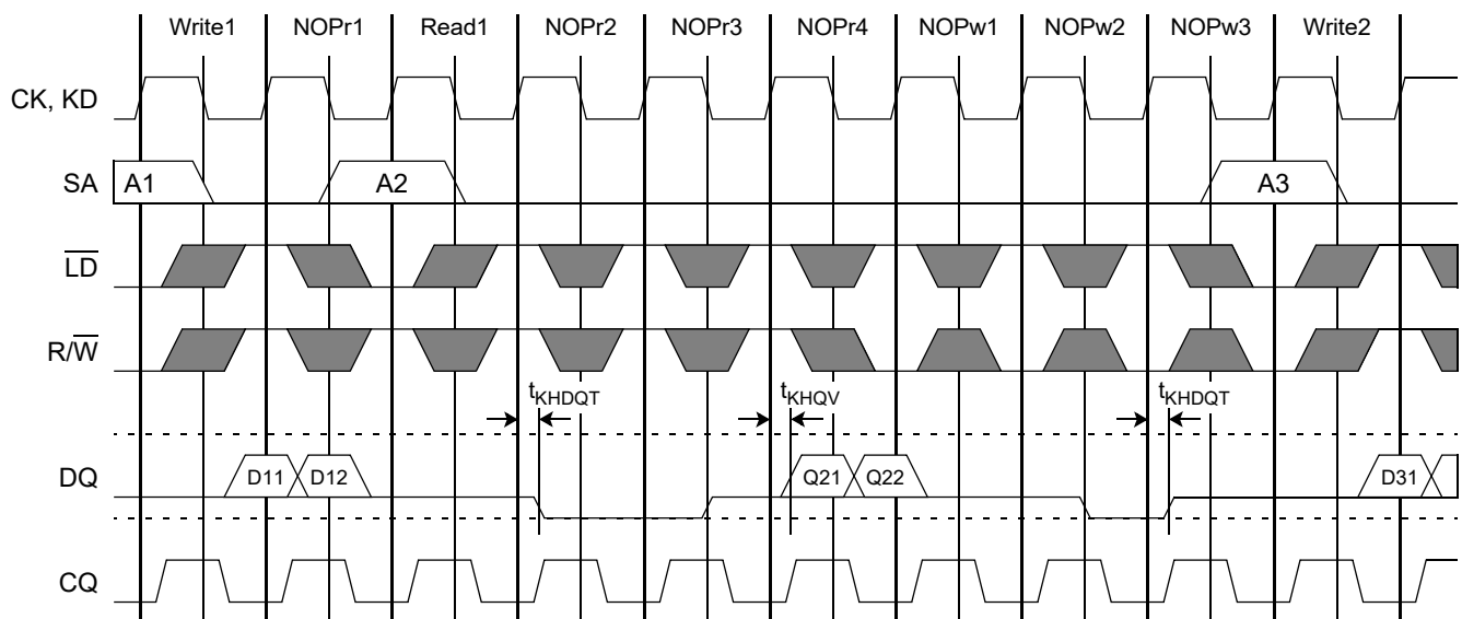
DQ ODT Control Timing Diagram
