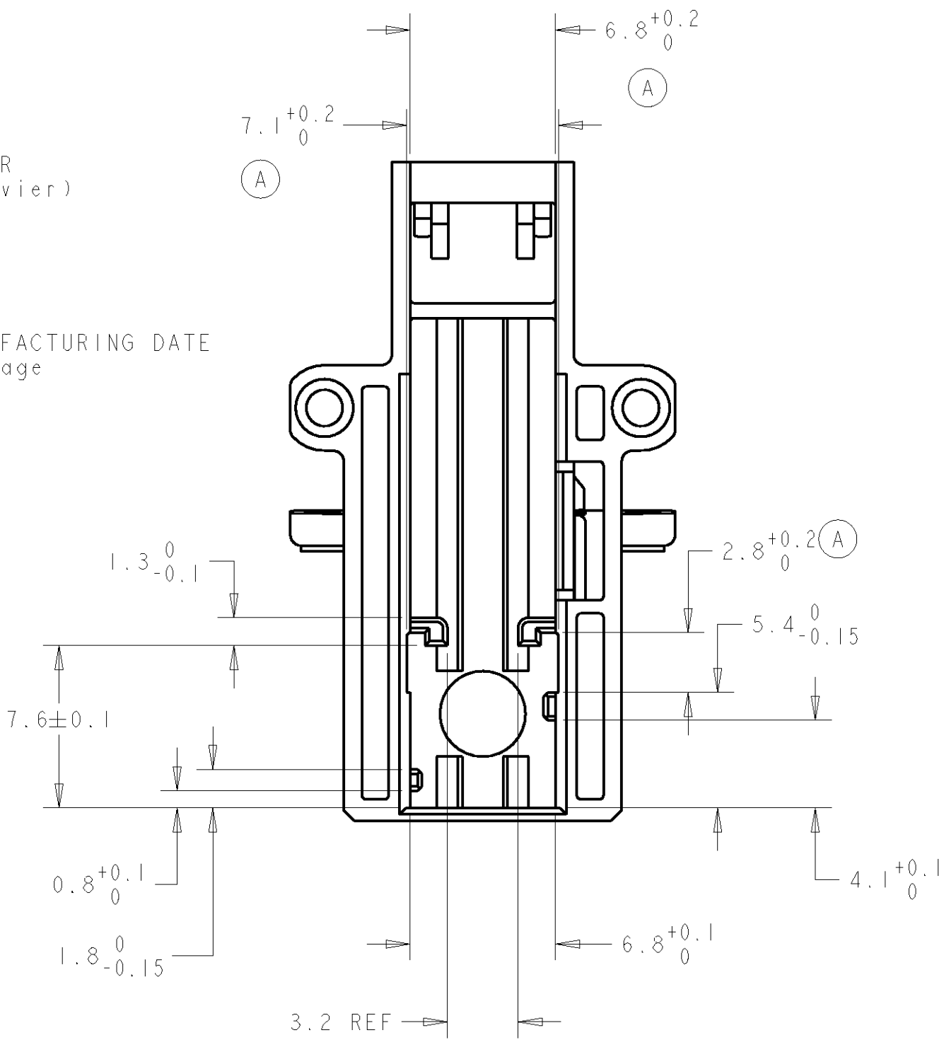
COUPE A-A
