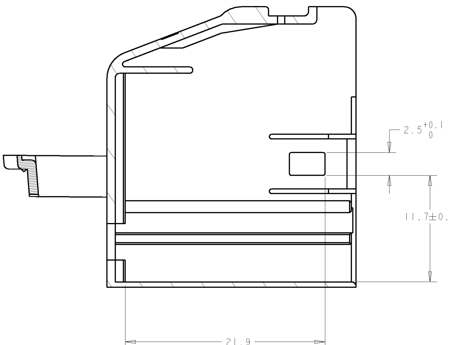
COUPE A-A
