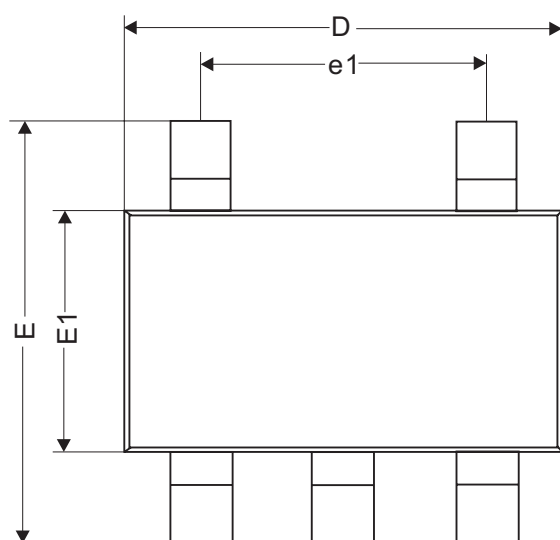
SOT23-5
