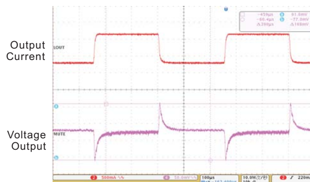
Load Transient Io=0-1A Vo=1.2V Vin=3.6V
