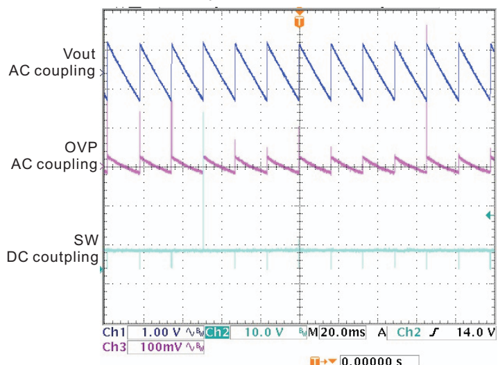
16. Open load
