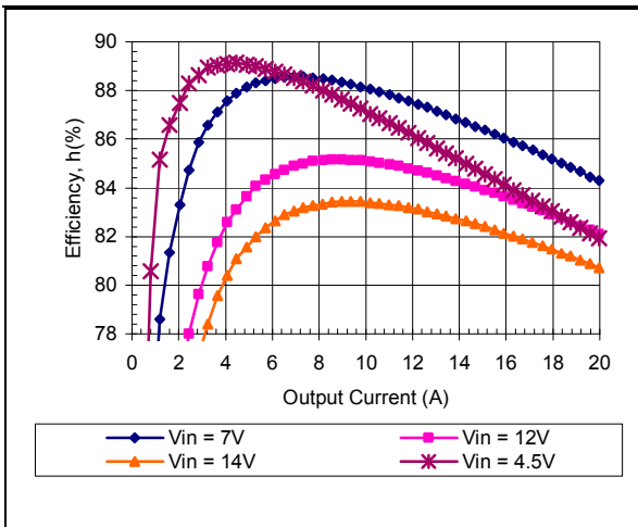
Vo = 1.2V
