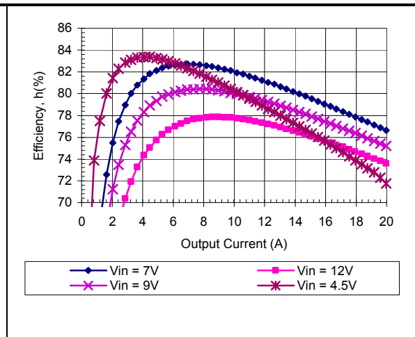
Vo = 0.7V
