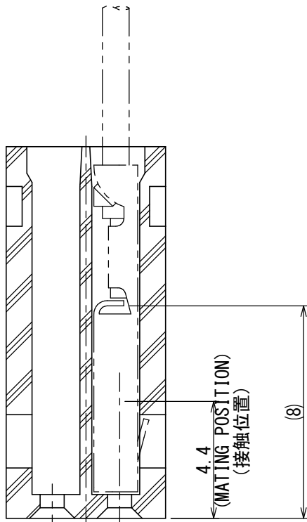
A-A (5 : 1)
