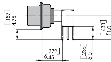
Connector with coaxial contacts FME001P... and signal contacts P5 Steckverbinder mit Koaxialkontakten FME001P... und Signalkontakten P5
