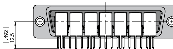
Connector with coaxial contacts FME018P... and signal contacts P5 Steckverbinder mit Koaxialkontakten FME018P... und Signalkontakten P5
