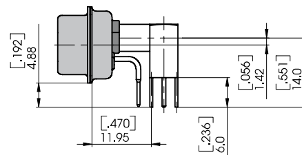
Connector with coaxial contacts FME018P... and signal contacts P5 Steckverbinder mit Koaxialkontakten FME018P... und Signalkontakten P5
