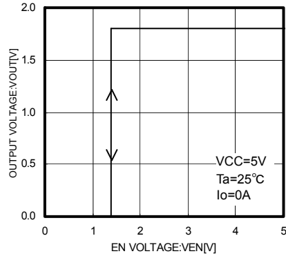
Fig.4 Ven-Vout
