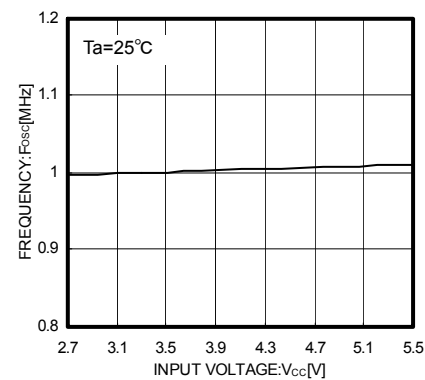
Fig.12 Vcc-Fosc
