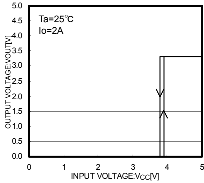
Fig.3 Vcc-Vout
