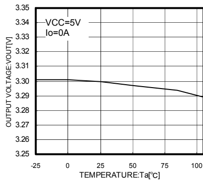
Fig. 6 Ta-VOUT
