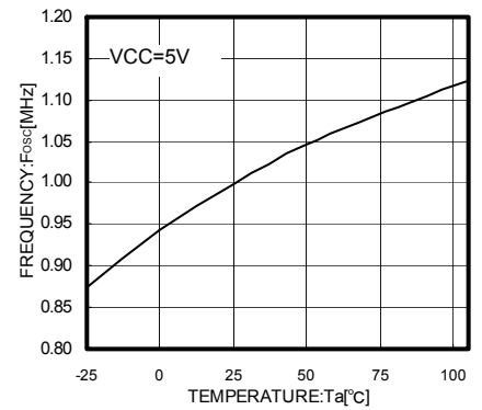
Fig.8 Ta-Fosc
