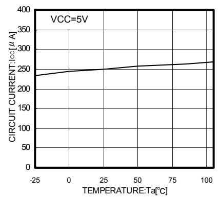
Fig.11 Ta-Icc
