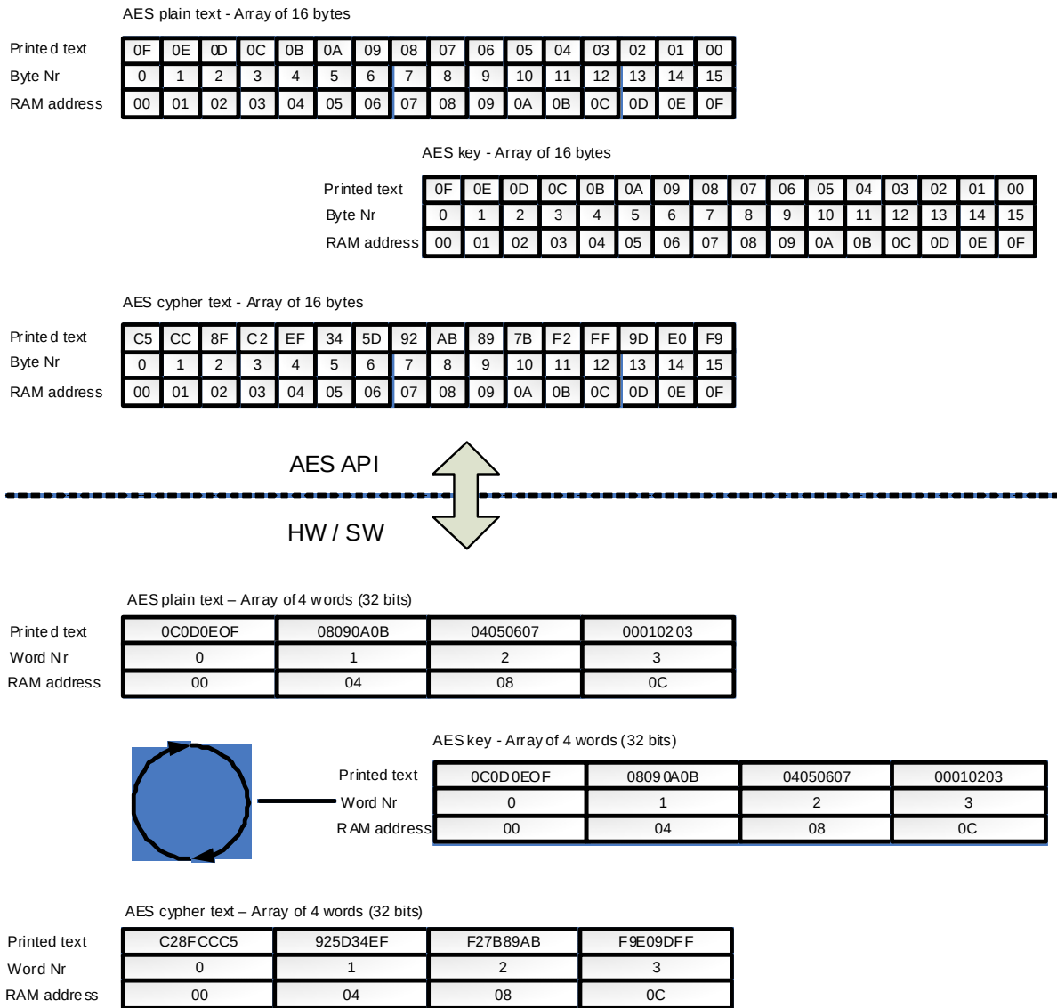
Fig 25. AES endianness
