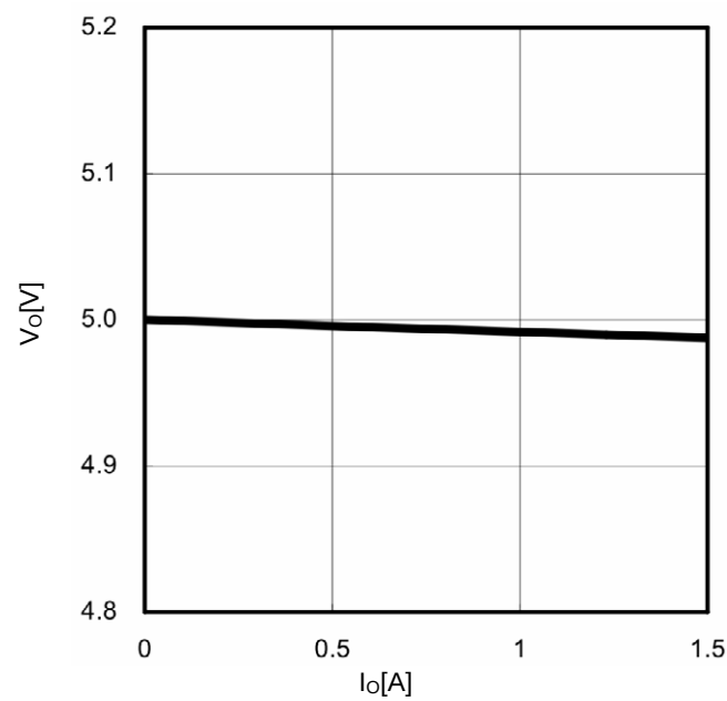
Fig.25 I_O - V_O
