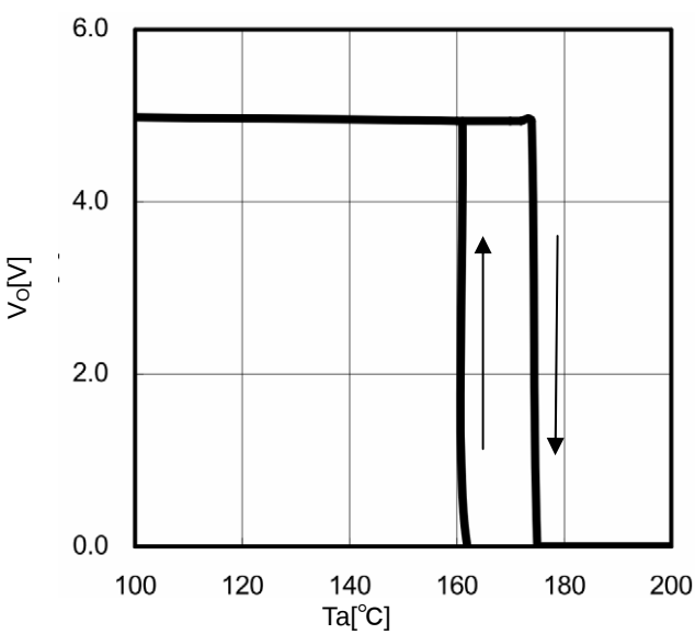
Fig.28 TSD ( I_o=0\text{mA} )
