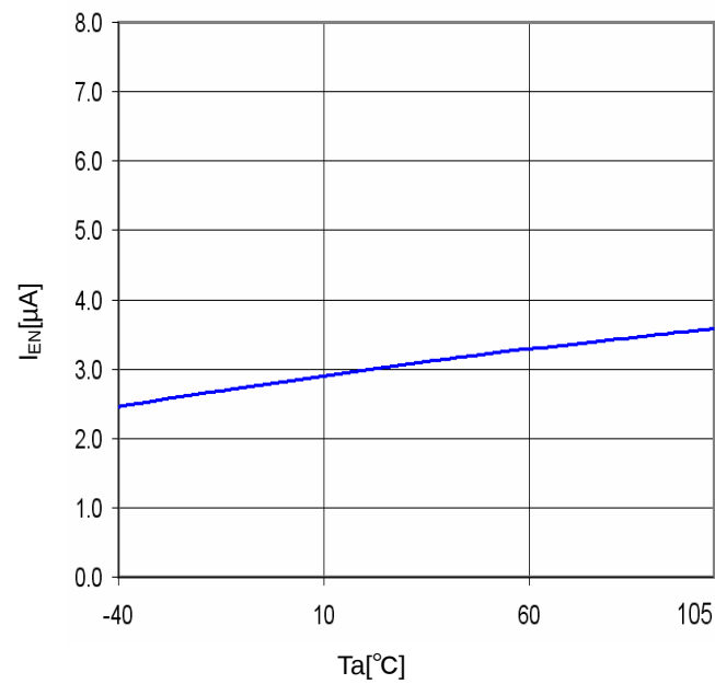
Fig.24 T_a - I_{EN}
