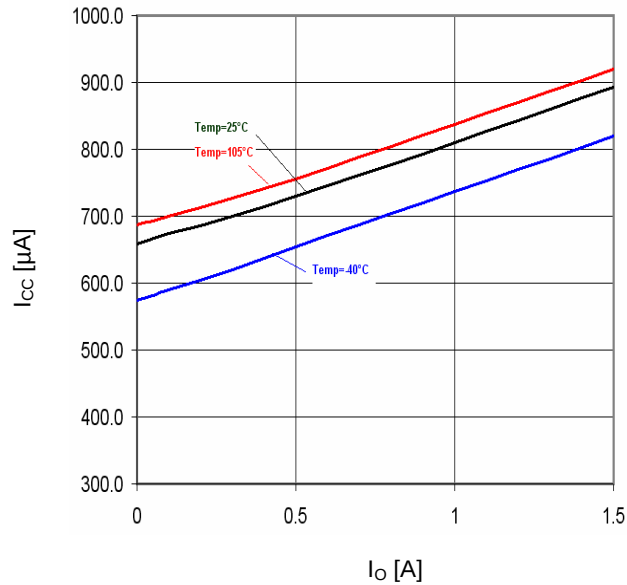
Fig.32 I_O - I_{CC}
