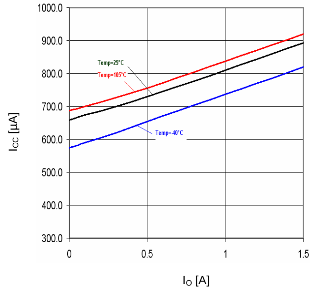
Fig.32 I_O - I_{CC}
